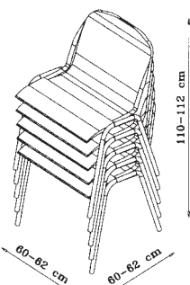
pila-pile 5 pz MC: 0,40
