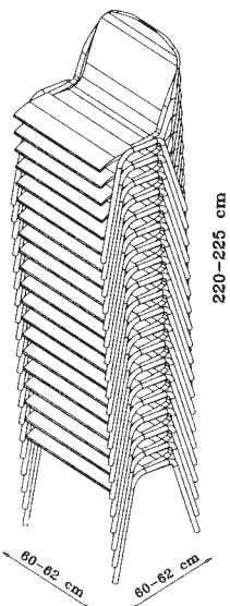
pila-pile 20 pz MC: 0,80
